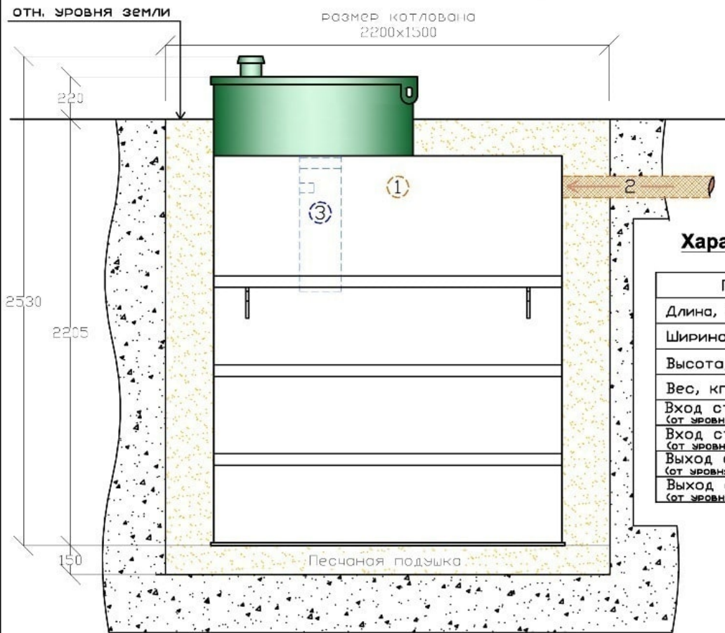
вид сбоку
