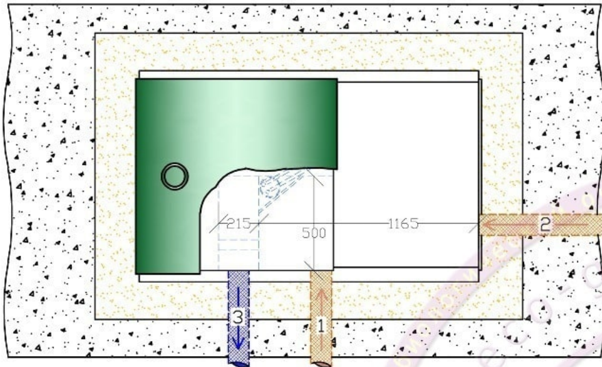
вид сверху
